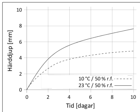
Diagram 1: Härdhastighet Sikaflex®-555
